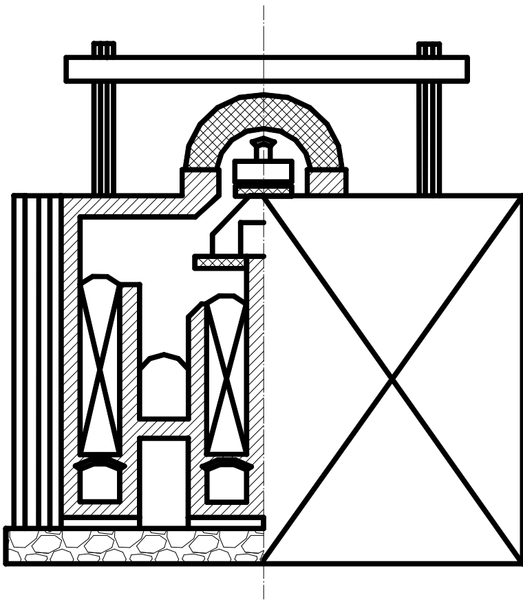
Типовая горшковая стекловаренная печь
