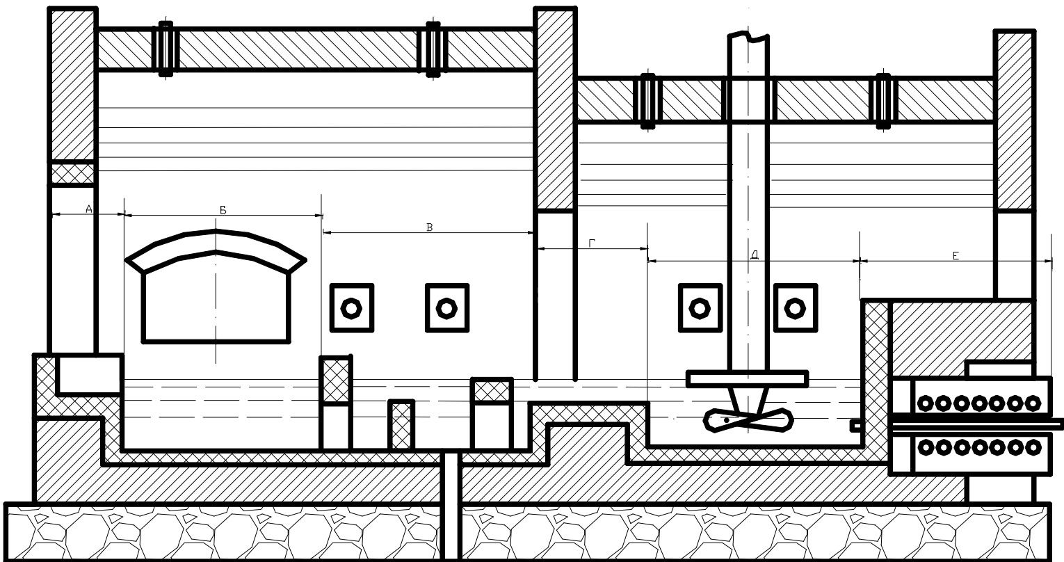
Ванная печь для варки оптического стекла
