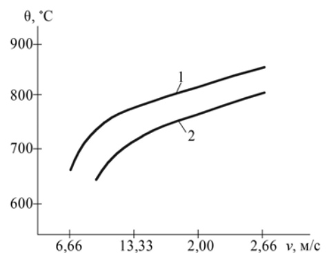
Рис. 4.7. Вплив швидкості різання на температуру різання при точінні звичайним різцем (1) та різцем із внутрішнім тепловідводом (2), різальна пластина ВК6; сталь 12Х18Н9Т; t = 0,5\text{ мм} ; S = 0,4\text{ мм/об}
