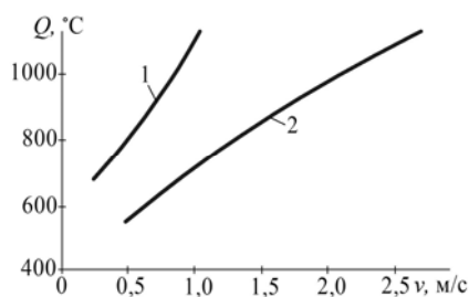
Рис. 3.5. Вплив подачі S (1) та глибини різання t (2) на температуру різання при чистовому точінні сталі 5XHM ( v = 1,8 м/с)
