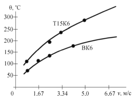
Рис. 3.18. Залежність температури від марки інструментального матеріалу при точінні склотекстоліту ( S = 0,21 мм/об; t = 1 мм)
