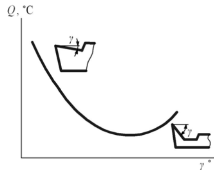
Рис. 4.4. Вплив переднього кута \gamma на температуру різання
