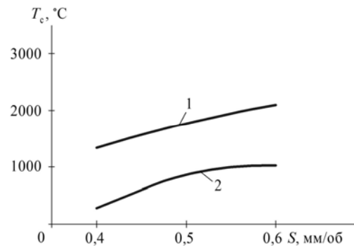
Рис. 3.15. Залежність температури спалахів T_c від швидкості різання: 1 – для пластичної ділянки контакту; 2 – для пружної; ( t = 0,4 мм; S = 0,22 мм/об)
