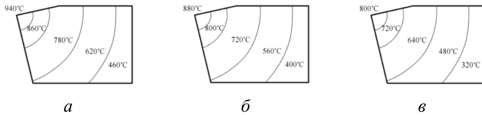
Рис. 3.2. Температурне поле різця із ПНТМ ельбор-Р при точінні сталей:
