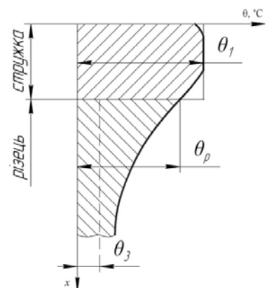
Рис. 1.4. Схема розподілу температури в системі «стружка-різець»: ( \theta_p – температура в площині дотику різця зі стружкою; \theta_1 – температура стружки в момент підходу до передньої поверхні різця; \theta_3 – початкова температура різця)
