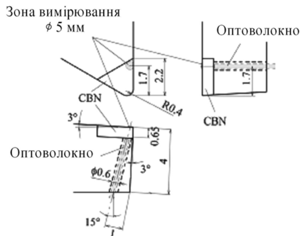
Рис. 2.4. Схема підводу оптичного волокна до різальної кромки інструмента
