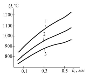
Рис. 3.4. Залежність температури різання від величини зносу різця по задній поверхні при точінні сталей 1 – ШХ15; 2 – 12ХН3А; 3 – 5ХНМ
