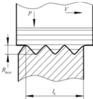
Рис. 3.11. Схема контакту
