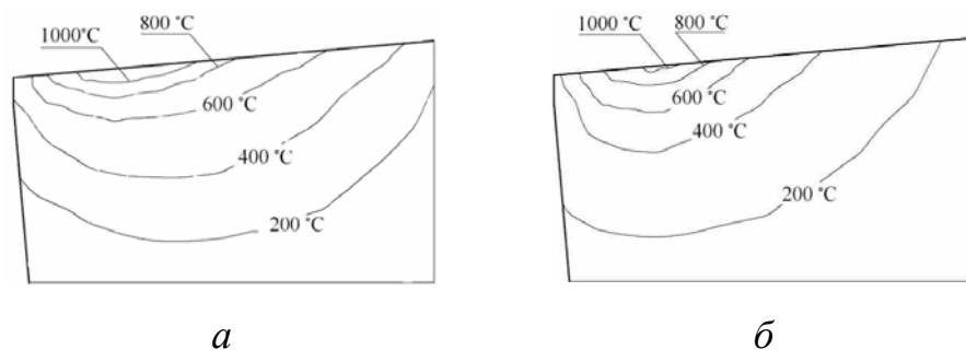
Рис. 4.14. Розподіл температури в різальному клині інструмента без покриття (а) та з покриттям TiN (б): v = 2,66 м/с; S = 0,3 мм/об; t = 1 мм
