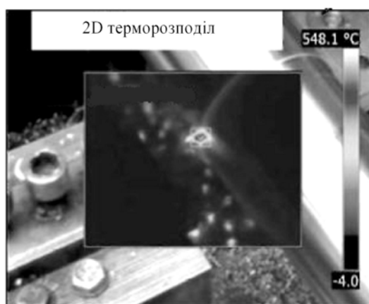
Рис. 2.5. 2D зображення розподілу температури в зоні різання отримане тепловізором.
