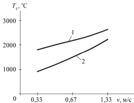
Рис. 3.14. Залежність температури спалахів T_c від подачі S : 1 – для пластичної ділянки контакту; 2 – для пружної; ( t = 0,4 мм; v = 1,0 м/с)
