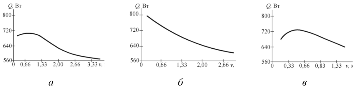
Рис. 4.17. Відносна інтенсивність охолодження зони різання водяним розчином соди та мастила при точінні різцем із твердого сплаву BK 8 – сталі 45 (а), 12X18H10T (б), титанового VT22 (в); ( S = 0,14 мм/об; t = 1,0 мм)
