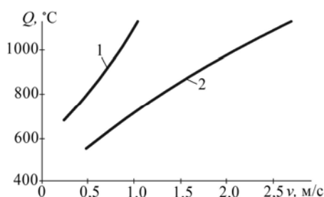
Рис. 3.3. Вплив швидкості різання на температуру при чистовому точінні ( S = 0,14 мм/об; t = 0,33 мм; h_z = 0,33 мм) сталі 5XHM (50-55 HRC), різцями із твердого сплаву T15K6 (1) і ПНТМ ельбор-Р(2)
