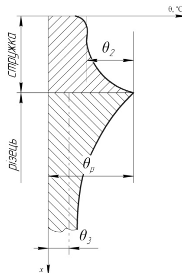
Рис. 1.6. Схема розподілу температури в системі «стружка-різець» при обробці чавуну
